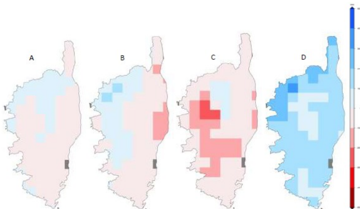
Figure 22 : Ecart de cumuls de précipitations moyens annuels (mm) en Corse relativement à la référence, pour le scénario RCP4.5, aux horizons proches 2021-2050 avec le modèle Aladin (A) ou WRF (B) et aux horizons lointains 2071-2100 avec le modèle Aladin (C) ou WRF (D).
